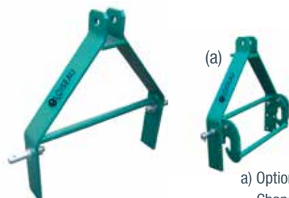
1 Attelage 3 points - Réf. RC-3P - 25 kg
